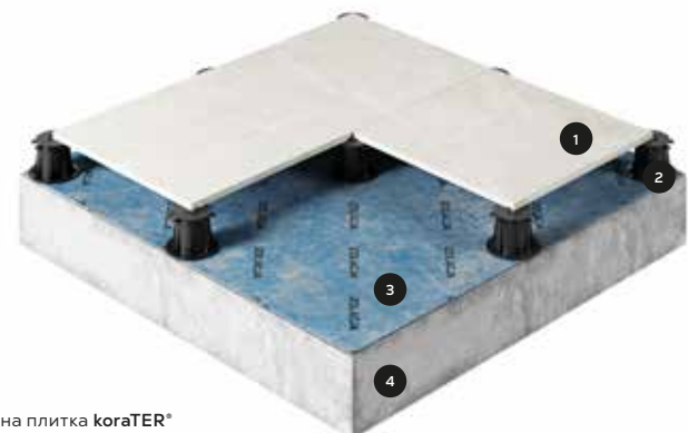
Укладання терасної плитки на регульовані опори
